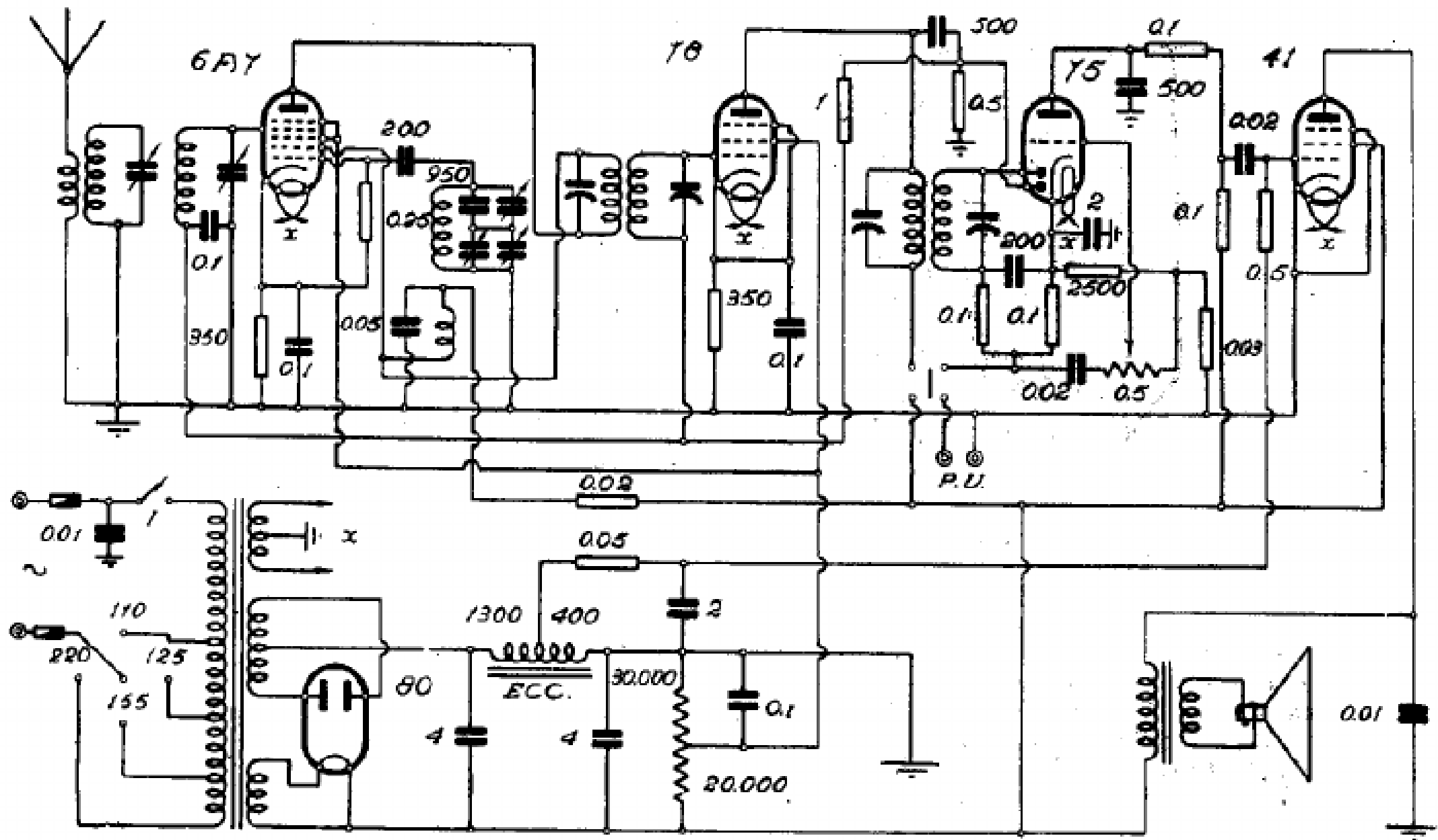
COMPAGNIA GENERALE DI ELETTRICITA' - MOD. « RADIORURALE »
